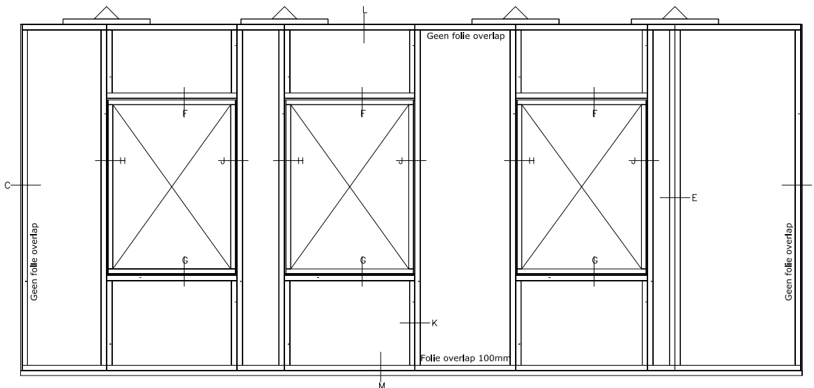
Figuur 3 Wand opgebouwd met Unidek SIPS
