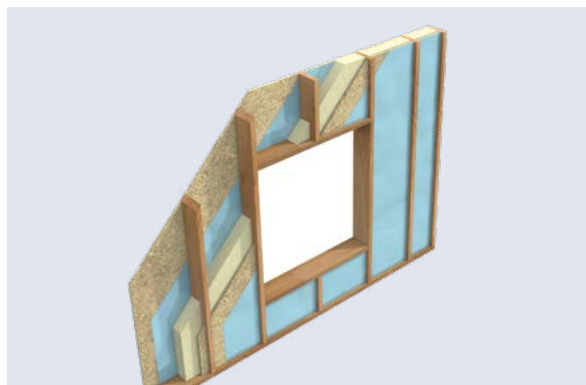
Voorbeeld van een HSB-gevelement
