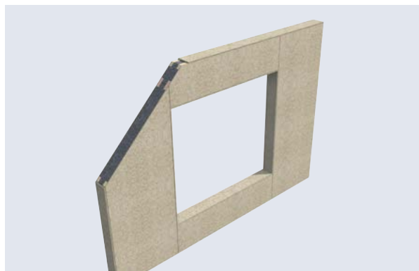
Voorbeeld van een Unidek SIPS samengesteld gevelement
